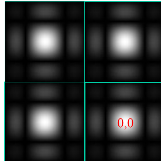
fftshift(fft2)
