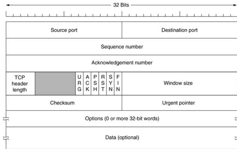
TCP Header.
