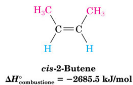
cis -2-Butene
