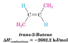
trans -2-Butene
