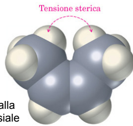
cis -2-Butene
