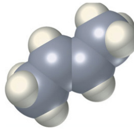
trans -2-Butene
