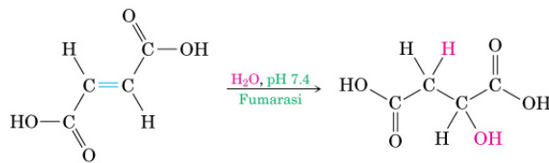
Acido fumarico
